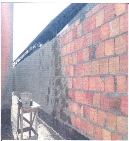
FOTO - 32 - ALVENARIA DE VEDAÇÃO DE BLOCOS CERÂMICOS FURADOS
