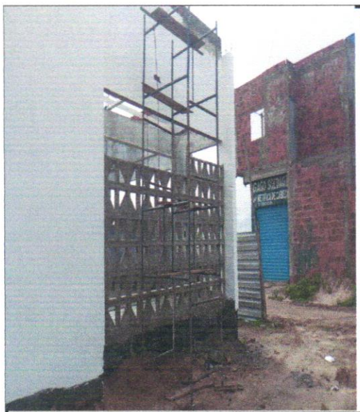
FOTO - 18 - APLICAÇÃO MANUAL DE MASSA ACRÍLICA EM PANOS DE FACHADA
